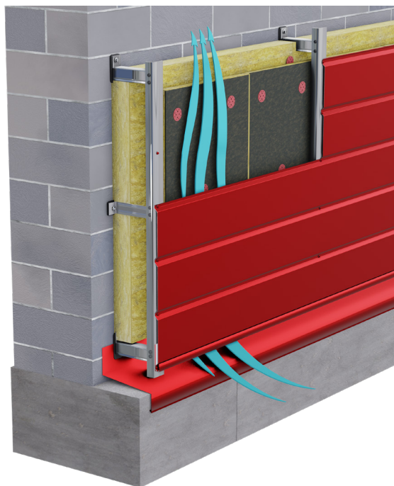
Фото 5. Система НВФ «Профіль СМАРТ-15»
